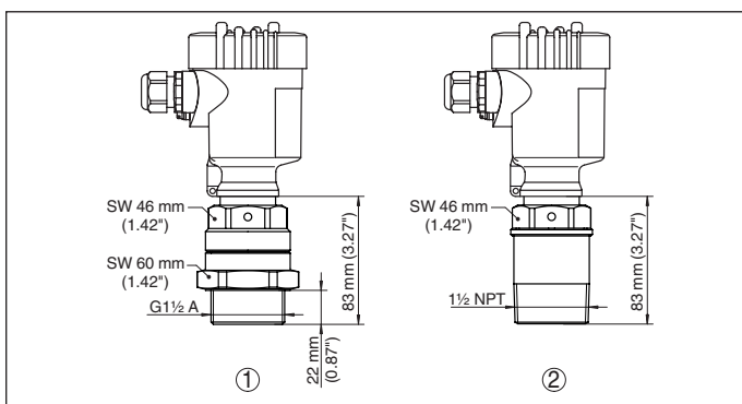
Fig. 21: VEGAMIP
