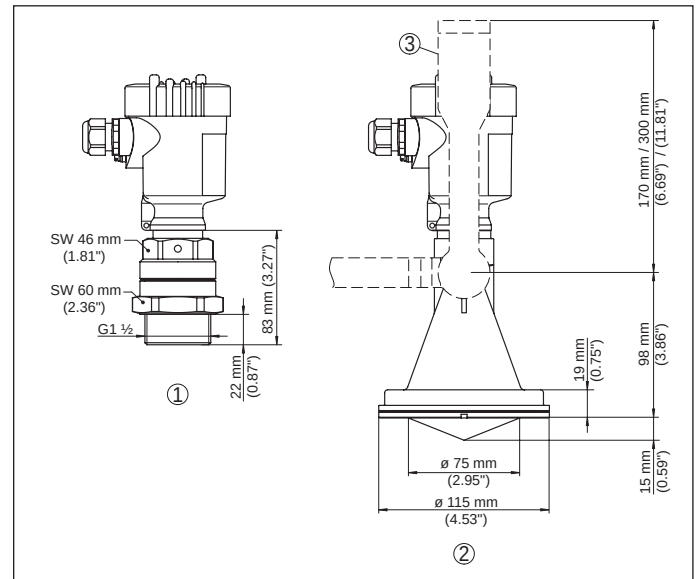
Fig. 22: VEGAMIP
