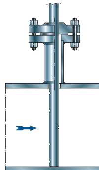
1F - 2F = Attacco al processo flangiato Dimensione flangia a richiesta. Process connection flanged Size flange to client request
