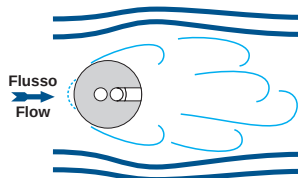
Sezione a profilo rotondo - Round section = T
